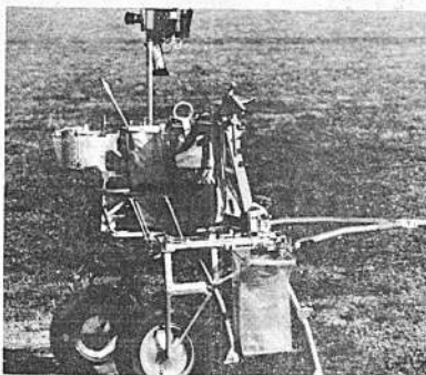
MESA DE TRABAJO PORTATIL. - Vista de cerca del transportador modular de equipo, apodado "litrakish", por su parecido, en su forma y manera de locomoción, a esta clase de carritos usados en el lejano oriente. Esa mesa de trabajo portátil, que utilizarán por primera vez los tripulantes del Apolo-14, tiene compartimientos para los herramientas de mano, lunares, cámaras, bolsa para almacenar muestras lunares y cables de película y un magnetómetro lunar portátil.
