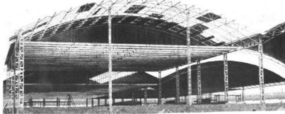
Una vista parcial de las obras civiles que actualmente se construyen en Río Seco para la Planta Industrializadora de Leche PIL, ciudad de La Paz. La casi totalidad de equipos y maquinarias ya se encuentran en el país y se tienen fijados para el mes de agosto la iniciación de trabajos.
