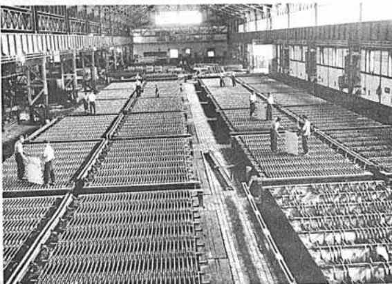
Proceso de electrolisis en la cuenca metalúrgica de Bor. Pertenecen a este conjunto metalúrgico minero las dos mayores minas de cobre yugoslavas.
