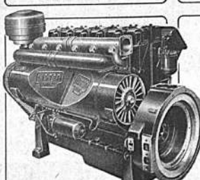
TIPO HR-6 88,5 HP-2.2000 RPM
