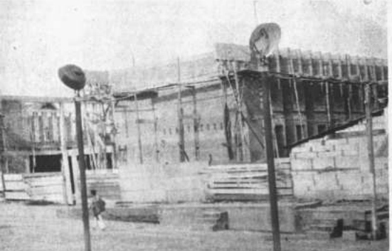
Construcción del Palacio de Justicia, Avance de la obra: 41,18 por ciento. Obra CORDENO.
