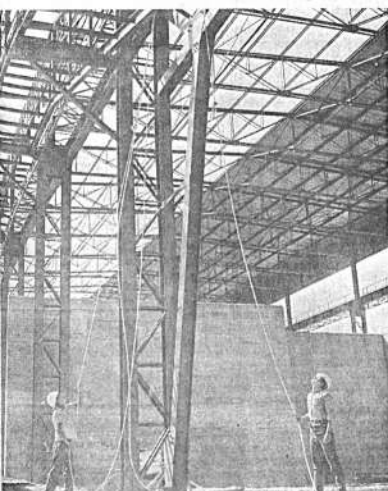
Así se levanta la estructura metálica de la fábrica de Cemento COBOCE en Cochabamba. Armado de estructura metálica interior del hangar de materiales, en Irap-Irap, Copinasta.
