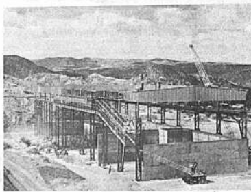
Hangar para recepción de la materia prima. Parte inferior del concreto armado. Parte superior, estructura metálica.
