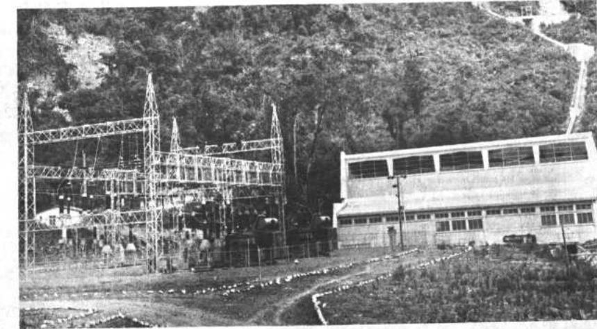
Proyecto Hidroeléctrico CORANI
