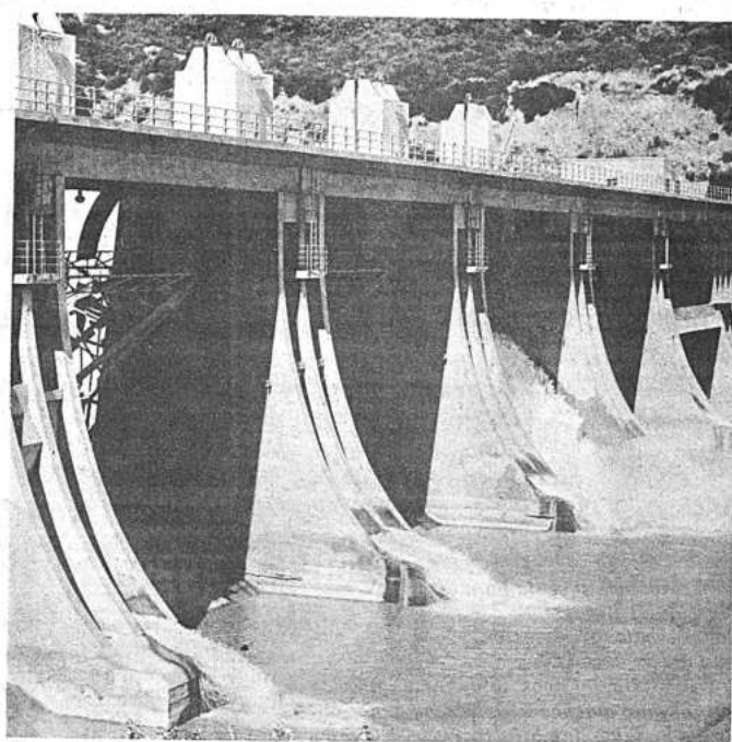
LA PRESA DE GANNANO, en la Provincia de Matera. Ubicada en el corazón de la comarca de Metapont, en Basilicata, constituye una de las principales obras de colonización efectuadas por la Caja del Mediodía en el cuadro de la política de Obras Públicas en favor de las regiones del Sur de Italia.
