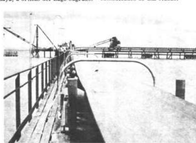
El muelle para cargar y descargar minerales y mercancías. Vista parcial de la correa transportadora que tiene una longitud de 325 metros y puede cargar 30 toneladas por minuto.
