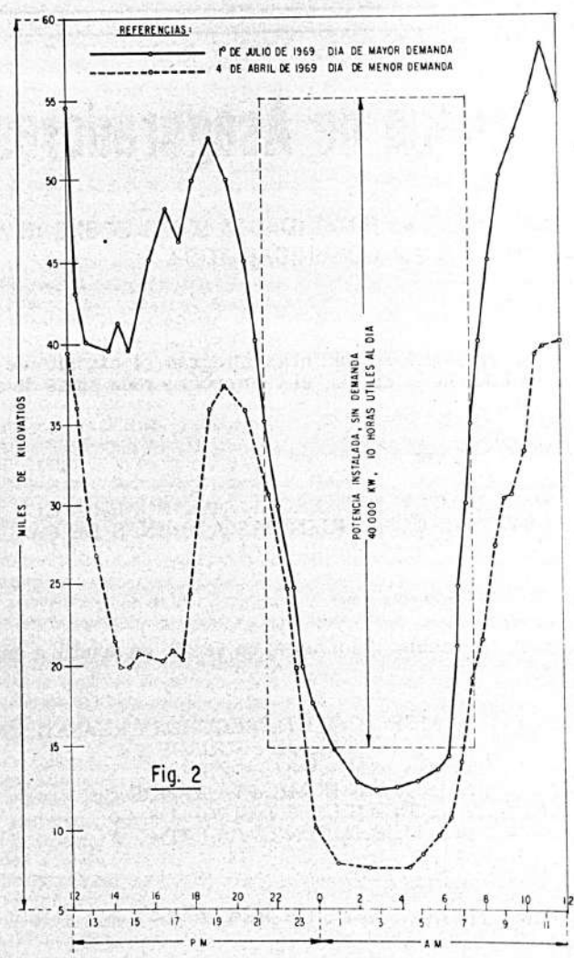
CIUDAD DE LA PAZ DEMANDA HORARIA DE ENERGIA
