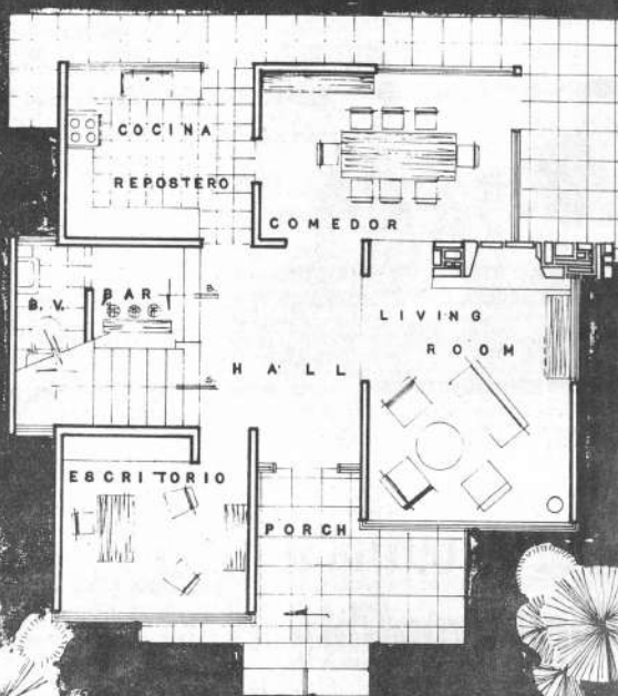
PLANTA BAJA
