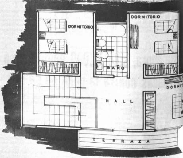
PLANTA ALTA
