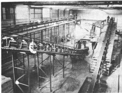
El BID ha contribuido a un programa para la rehabilitación de la minería estibadora del país. En la fotografía se aprecia la transportadora de minerales que funciona en el ingenio Sink and Float de Catavi.
