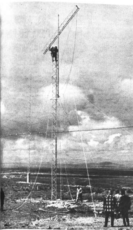
Técnicos de la Empresa Nacional de Telecomunicaciones, instalando las antenas logarítmico-periódicas en la zona de Achacicala.
