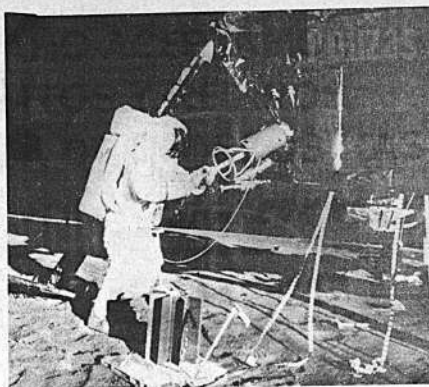
DEL ALUNIZAJE DEL APOLO-12. Generador atómico en la Luna un recipiente cilíndrico de combustible radioactivo es extraído de un compartimento aislado, asegurado al módulo lunar "Intrepid", por uno de los astronautas de la nave Apollo-12.
