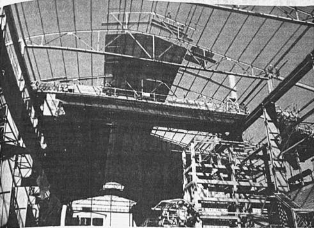
GIGANTESCA OBRA ESTA POR CONCLUIR. La fundición de estaño que se está construyendo en Vinto empezará a funcionar dentro de un año. Las primeras pruebas se realizarán a partir de mayo próximo. La obra, una de las más grandes emprendidas hasta ahora por el país y el comienzo de la gran industria metalúrgica nacional, habrá demandado, al concluir su primera etapa, una inversión aproximada de doce millones de dólares. La fotografía muestra la magnitud de las instalaciones. - Amba, pequeños como hormigas, algunos obreros trabajan. (Infot. páginas centrales)
