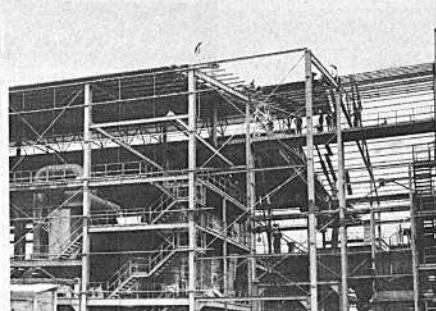
Vista parcial de una de las estructuras metálicas de la fundición de estaño que se está construyendo en Vinto De acuerdo a los informes técnicos, la planta será una de las más modernas de Latinoamérica.
