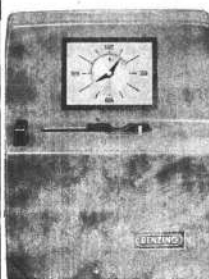
KA 1500 Accionamiento por mecanismo de resorte y mecanismo de relajación de áncora.
