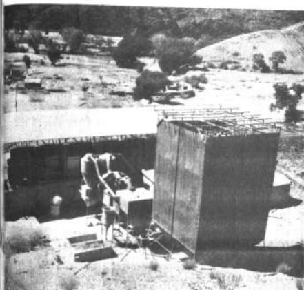
La aparentemente complicada maquinaria de la fundición Artola. Se diseñó y fabricó en Tupiza.
