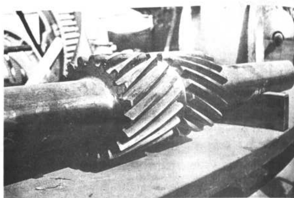
Los diferentes piezas de maquinaria pesada, que son fabricadas en los talleres propios de Comibol, concitaron la atención del público en la VI Feria de Santa Cruz. En el gráfico, un engranaje helicoidal para molino de minerales.
