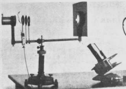
Fotocoagulador en el que se utiliza el sol como fuente de luz.
