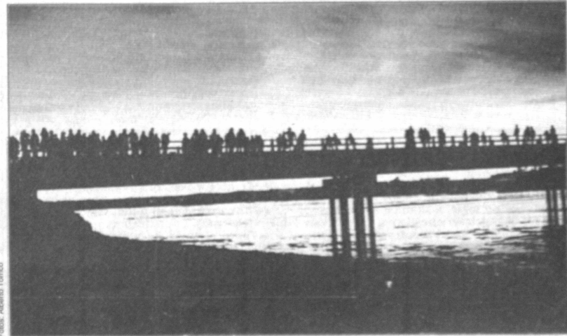
Científicos, turistas nacionales y extranjeros se congregaron en varias partes del te- rritorio nacional, para observar el sobrecogedor espectáculo de la "muerte del Sol". Las fotografías de abajo, en Huachacalla, muestran la diferencia entre el amanecer y el momento del oscurecimiento. Arriba, a la izquierda, la corona radiante o de dia- mante tomada con lente normal en la región de Sevaruyo.
