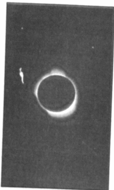
La muerte del Sol Momento culminante del eclipse cuando la Luna cubre totalmente al Sol.
