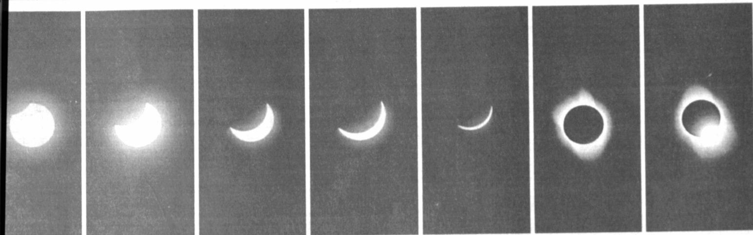
Espectacular secuencia del eclipse total de Sol en la zona de Sevaruyo.
