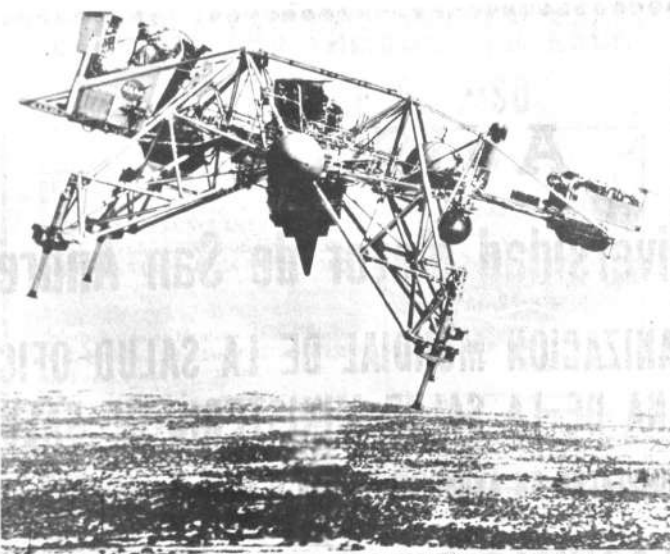
El piloto de pruebas Dan McIllick realiza un aterrizaje lunar simulado con un vehículo de investigación de aterrizaje en la Luna, en el Lago Seco Rogers, en California. El aparato que corce de alas, tiene dispositivos que compensan las diferencias atmosféricas y de gravitación entre la tierra y la Luna.
