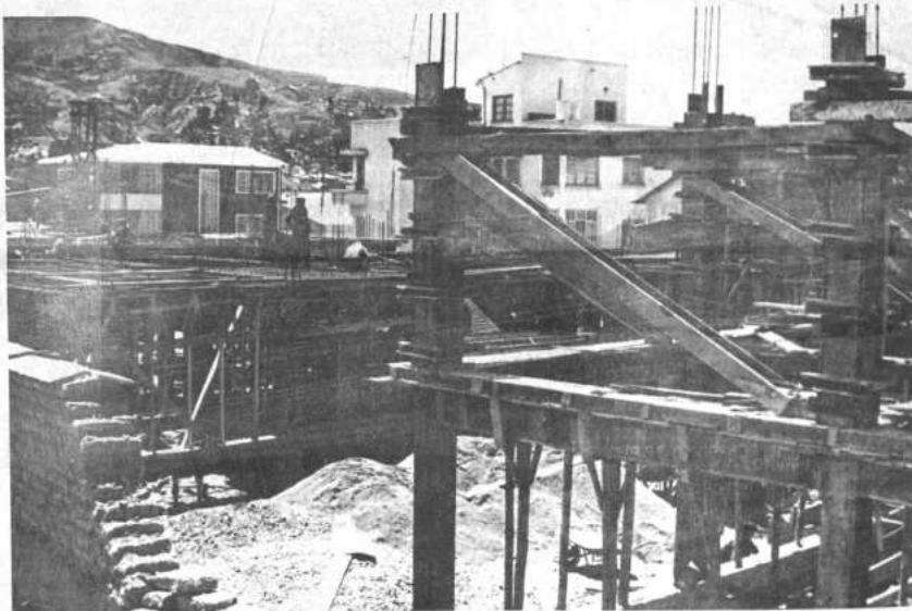
Los trabajos de construcción de tres edificios multifamiliares que se ejecutan en la avenida Busch, están bastante avanzados. En la fotografía se ven las estructuras de cemento.
