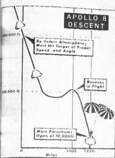
Este diagrama muestra la trayectoria de la Apollo-8 en su ingreso a la atmósfera terrestre y descenso en el Pacífico. (AP RADIOFOTO)
