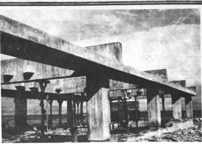
ESTRUCTURA DEL DEPARTAMENTO DE FÍSICA. — Construido a base de hormigón armado, consistente en pilares colocados cada diez metros que definen recintos de 100 metros cuadrados cubiertos por techos piramidales. Estos recintos podrán ampliarse en el futuro, cuando menos por dos costados de acuerdo a las futuras necesidades.
