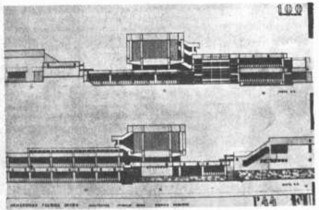
BIBLIOTECA DE LA FACULTAD DE INGENIERIA. — La fotografía muestra una elevación de la Biblioteca de la Facultad de Ingeniería que se levanta sobre un lecho de cantera aprovechando para jardín y como espacio de esparcimiento.
