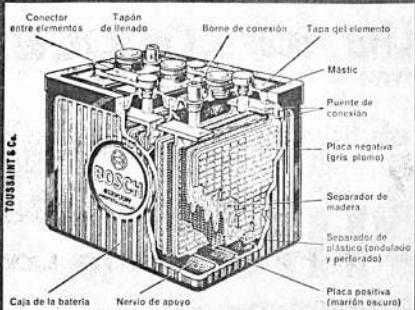
Fig. 1 Estructura de una batería de plomo Bosch para vehículos de motor
