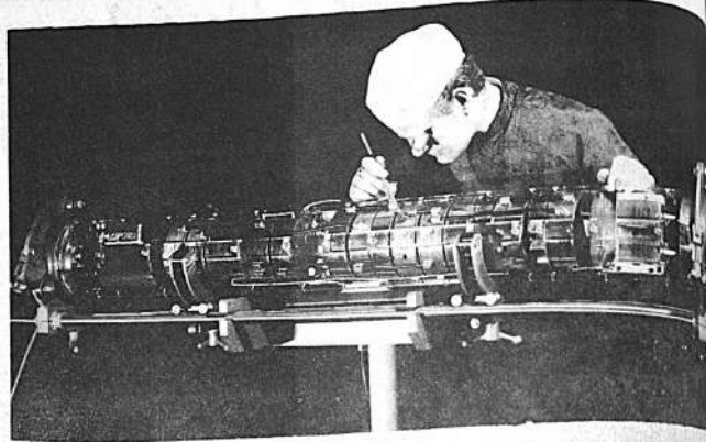
Un ingeniero inspecciona una cápsula de repetición transistorizada en la Standard Telephone and Cables de Londres. Estos repetidores forman parte, junto con cables y equipo para terminales, del contrato por 10,800,000 dólares por 1,800 km. de cable submarino entre Italia y España, donde se comunicará con el cable TAT que unirá España con Estados Unidos en 1976. El complejo de comunicaciones costará 96 millones de dólares y revolucionará las comunicaciones entre el sur de Europa y los EE.UU.
