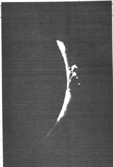
Una protuberancia solar
