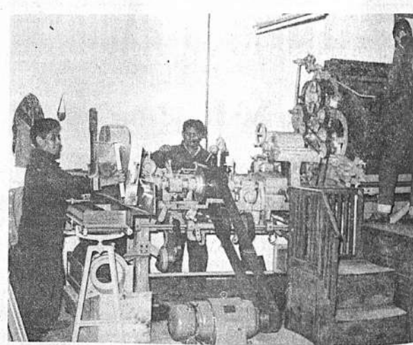
El equipo cigarrero instalado en Santa Cruz de la Sierra tiene capacidad para elaborar 400 cajetillas al mes en directiva combinación con el resto de las máquinas de la fábrica. La unidad cigarrera en plena producción del cigarrillo ORIENTAL con tabaco negro.
