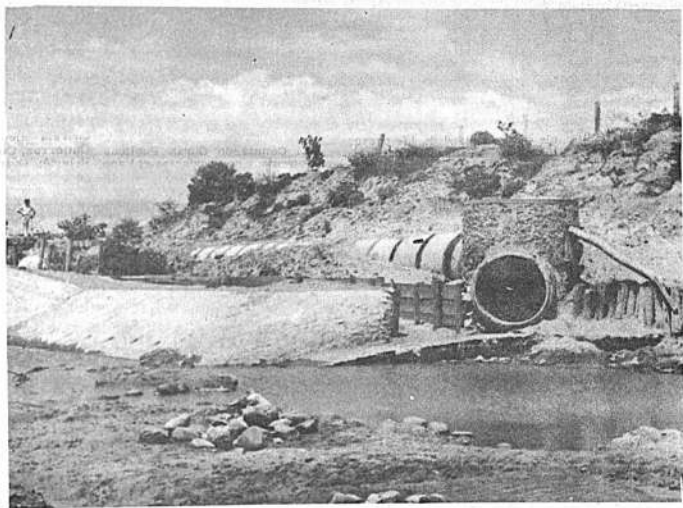
Aquí, el canal de Isuta ubicado al noroeste de la ciudad, desemboca el sistema de alcantarillado de Santa Cruz de la Sierra. Actualmente está en servicio el alcantarillado pluvial faltando la construcción de la planta de tratamiento para el funcionamiento del cloacal.
