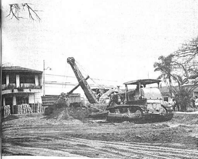
Santa Cruz de la Sierra, día tras día, va adquiriendo una nueva fisonomía en mérito al trabajo que realiza el Comité Departamental de Obras Públicas. Maquinarias pesadas van venciendo los desniveles de las calzadas para proceder posteriormente a su enlosamiento. Hasta el momento se han colocado 250.000 metros cuadrados de losetas.
