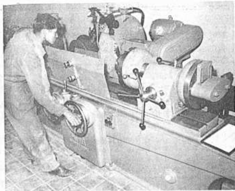
Moderna máquina utilizada en la rectificación de cigüeñales y realización de otros técnicos.
