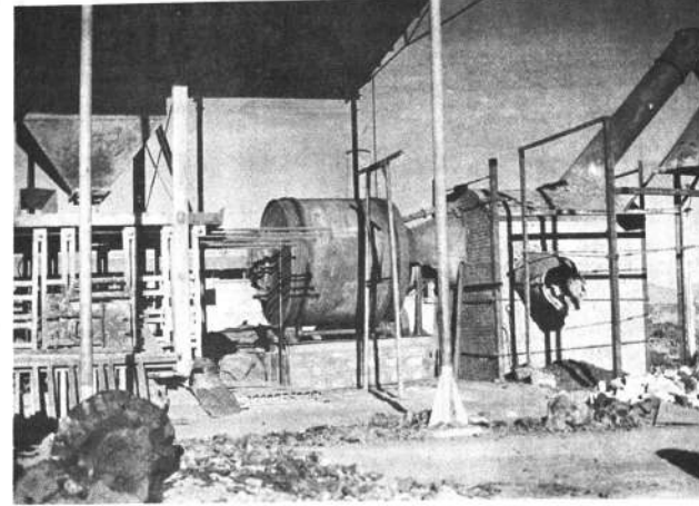
Planta de volatilización de minerales.
