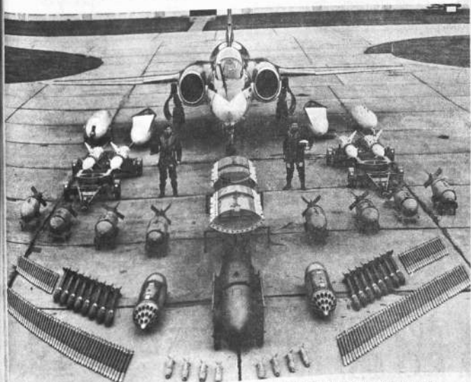
Un pedido de 26 "Buccaners", aviones de ataque, para la RAF por unos 62 millones de dólares acaba de recibir la Hawker Siddeley de Gran Bretaña. El "Buccaner" es un avión que opera a baja altitud al que vemos aquí con su carga típica, bombas, tanques extra de combustible, y porta cámaras fotográficas. Puede llevar un proyectil nuclear o el proyectil anglo-checo y porta cámara fotográfica. Los 26 "Buccaners" con otros ya en servicio función Myster entre a tierra, de gran precisión. Los 26 "Buccaners" con otros ya en servicio
