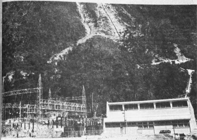
La Planta Hidroeléctrica de Corani, inaugurada recientemente, es el proyecto más grande de electricidad que ha construido la Empresa Nacional de Electricidad conjuntamente con el Banco Interamericano de Desarrollo, dentro de los programas de la Alianza para el Progreso. La producción eléctrica de Corani ya beneficia a la ciudad de Cochabamba y facilitará la industrialización de los Departamentos de Oruro y Potosí.
