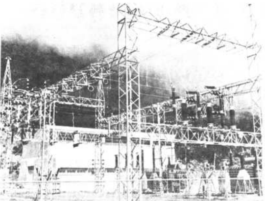
Subestación de la Planta Central de Hidrocarburos de Corani.
