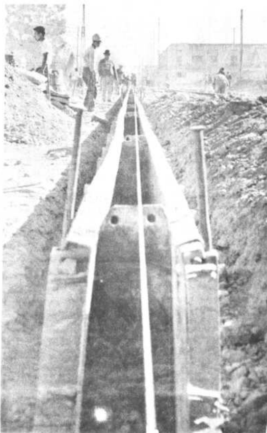
En la Av. San Martín se aceleran los trabajos para la construcción de cintos de acero.
