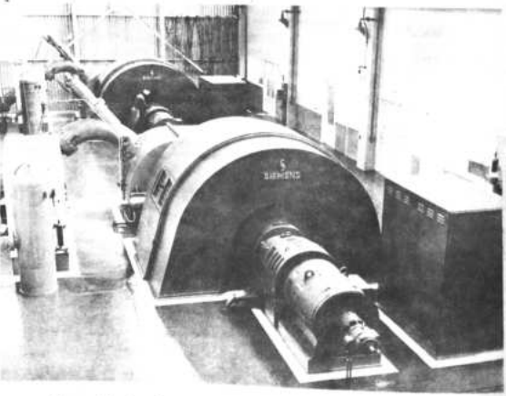
Dos unidades de Generación en la casa de máquinas de la Planta Hidroeléctrica de Corani.
