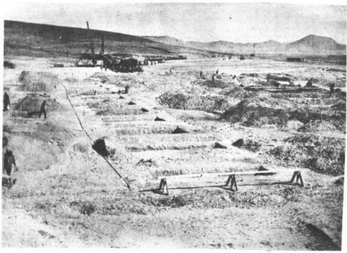
Aceleradamente se trabajan en Vinto, a 8 kilómetros de Oruro, las obras preliminares para las instalaciones de los hornos de fundición de minerales, dentro del contrato Klockner.
