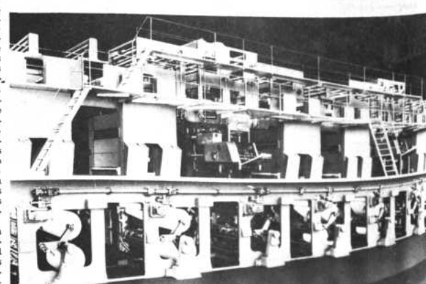
Rotativa M.A.N. para periódicos que combina la impresión en relieve con el offset en relieve.
