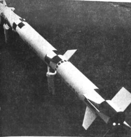
Cohete antibalístico denominado "Spartan", que fue sometido a prueba con todo éxito en Kwalein, en los islas Marshall. La configuración externa del cohete, de 16,7 metros de longitud, con sus etapas, fue por primera vez exhibido en la planta McDonnell Douglas, de California. Tiene un alcance de aproximadamente 650 kilómetros.
