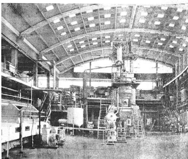
Vista general de la planta con la instalación del equipo automático "Mazzoni".
