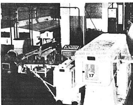
Troqueladora automática sincronizada para los diferentes formatos de jabones comunes y de tocador.
