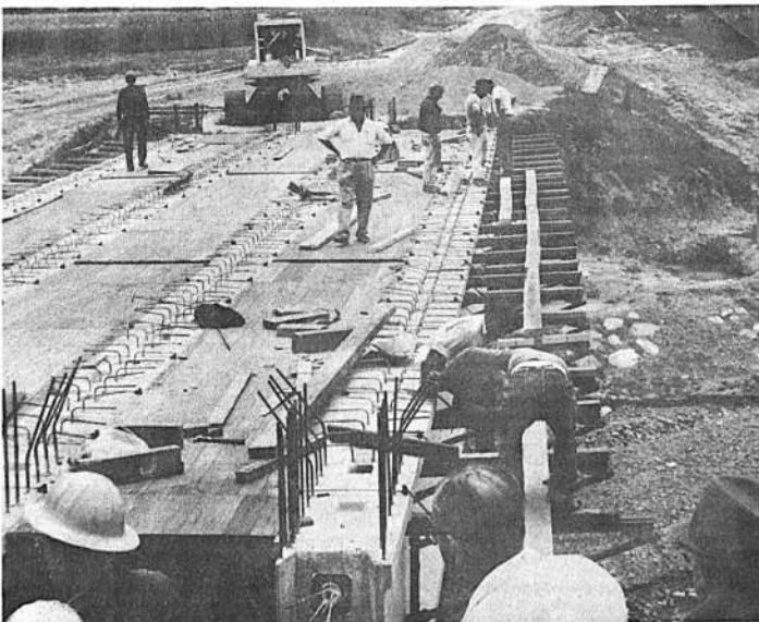
Uno de los puentes que se construyen en Cochabamba, dentro del proyecto carretero uno y cuatro. Estos puentes, que tienen una capacidad de 20 toneladas, cuestan de 160.000 dólares a 80.000 dólares. También en esta fotografía se puede observar que los obreros carecen de ropa de trabajo.]
