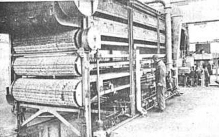
Tres aspectos de la fabricación de fósforos: Una laminadora (arriba) prepara el material que será cortado hasta convertirse en millones de palitos. Una máquina (centro) recibe los palitos; un extremo de cada uno de éstos será bañado con fósforo. Los palitos (abajo) salen en cajitas que llevan etiquetas con paisajes de cada uno de los Departamentos geográficos del país.
