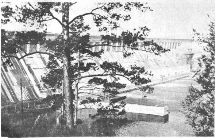
En Siberia, en el río Angará ha terminado la construcción del gigante energético mayor del mundo la central hidroeléctrica de Bratsk, de una potencia de 4,1 millones de kilovatios. La central produce 22,6 mil millones de kilovatios/hora al año. Los aguas del Angará ponen en acción turbinas de 225 y 250 mil kilovatios de potencia. La extensión de las líneas de transmisión de energía, de una tensión de 220 y 250 kilovoltios, es de unos tres mil kilómetros. Las empresas industriales y obras de Siberia recibirán millones de kilovatios de energía eléctrica barata.
