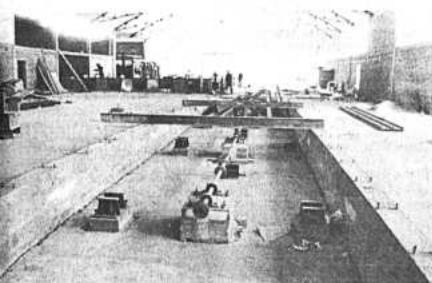
Vista del amplio galpón con la laminadora al fondo.
