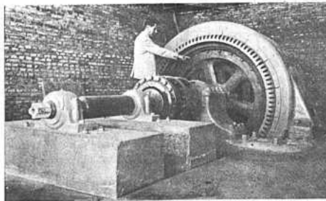
MOTOR GE de 1.000 HP de fuerza con un peso de 20.000 Kg.
