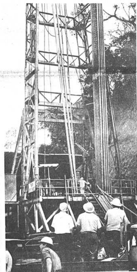
Este es el pozo dirigido No. 8 mediante el cual se encontrará el descontrol del No. 7 subterráneamente. El trabajo debe realizarse con una precisión ya se trata de encontrar a 1,500 metros de profundidad una apertura de más o menos 9 pulgadas de ancho.
