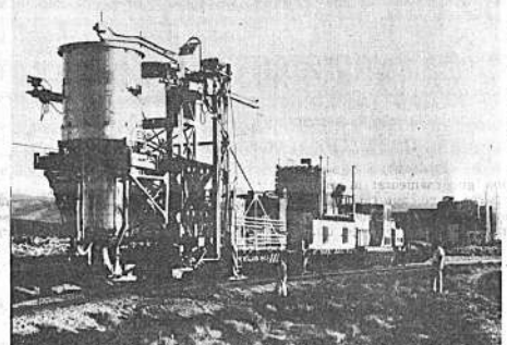
Un motor nuclear sin combustible, transportando hasta el lugar de pruebas en Nevada. El motor es una versión adelantada que será empleado en investigaciones para vuelos de larga distancia a planetas lejanos.
