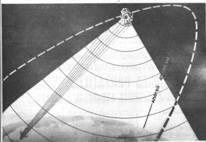
Esquema que muestra la exposición de la Tierra por el satélite "Molnia-1".
