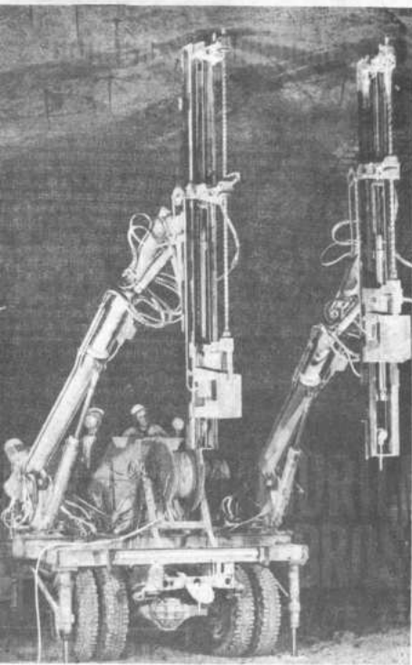
De una agilidad realmente acrobática es un nuevo "robot de aludrar", desarrollado por una conocida fábrica en la República Federal de Alemania. El aparato portátil con sus brazos orientables es utilizado en la construcción de túneles y de galerías de minas. En el calado de agujeros de mina y de acople abrevia el tiempo de trabajo a una fracción del que hasta ahora necesitaba. Los gigantescos husillos portabrocas penetran fácilmente hasta en las rocas más duras. Lo que ayer fue todavía trabajo pesadísimo, muchas veces de larga duración, lo determinará de ahora en adelante el robot en un centésimo.
