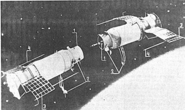
Esta ilustración gráfica da una idea de la forma en que se produjo el acoplamiento automático de dos naves espaciales soviéticas la semana pasada. Las naves no estaban tripuladas. (AP Wirephoto)
