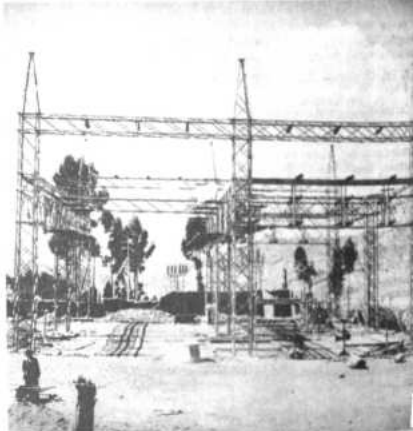
Estructura metálica instalada en Rossasani para la operación cómoda y segura de las líneas de transmisión de 115.000 voltios.
