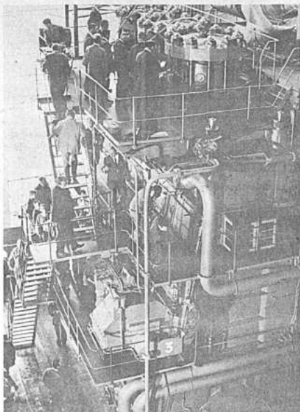
MOTOR DE GRAN ALTURA. Este es el motor Diesel más grande del mundo que se encuentra desde hace poco en el puesto de ensayo de la Maschinenfabrik Augsburg-Nürnberg. Tiene una altura de 14 metros, tres cilindros y una potencia de 12.000 cv. Se lo puede agrandar en diez cilindros. Las ventajas de la gigantesca construcción son su rentabilidad y su fácil entretenimiento que recomiendan montarla, incluso en los petroleros más grandes.
