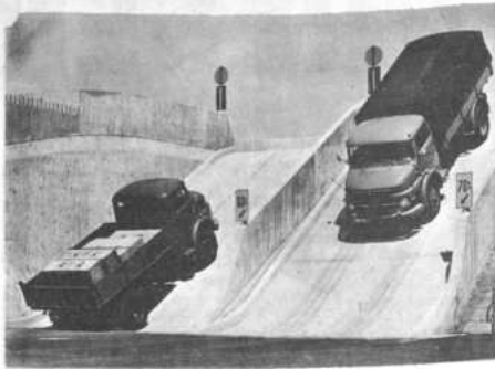
Una "carretera de montaña", de pruebas, fue recientemente inaugurada en Alemania Federal por una fábrica de automóviles. En los trayectos de 1,5 Km. de largo, los vehículos son expuestos a toda clase de pendiente vigilados por sistemas de medición y control. El camión cargado salvó la pendiente del 60 por ciento, el patrón cuando en el declive del 70 por ciento fue sabiamente frenado y dio marcha atrás.
