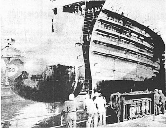
Con este petroero de 190.000 toneladas, en vías de construcción en Kiel, en la costa del Mar Báltico, tendrá una longitud de 323,7 m, mientras que el dique mide sólo 310 m. se tuvo que montar la proa posteriormente en el casco ya flotante. Los expertos opinan que según este método será posible construir buques más grandes aún en los diques secos tradicionales.
