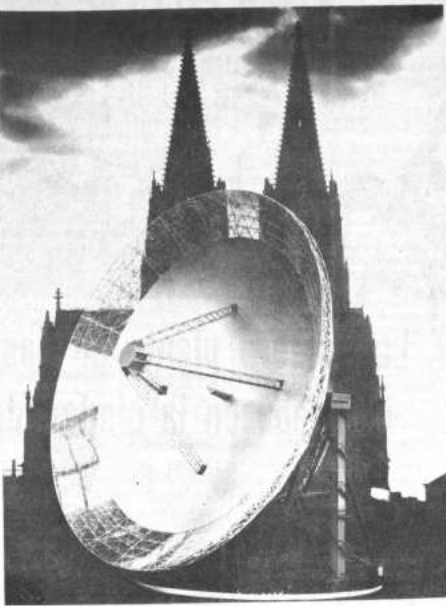
Gigantesco radar telescópico que será instalado en las montañas de Ellet (Alemania Occidental) en 1969. Este radar que tiene un espejo parabólico de cien metros de altura, pesa aproximadamente 2,800 toneladas, su tamaño es comparado en la fotografía con la Catedral de Colonia (que se ve al fondo) y está sostenido sobre una base circular de 64 metros de diámetro. Permitirá a los astrónomos realizar investigaciones de las radiaciones en el universo, que se producen a millones de kilómetros de la Tierra.
