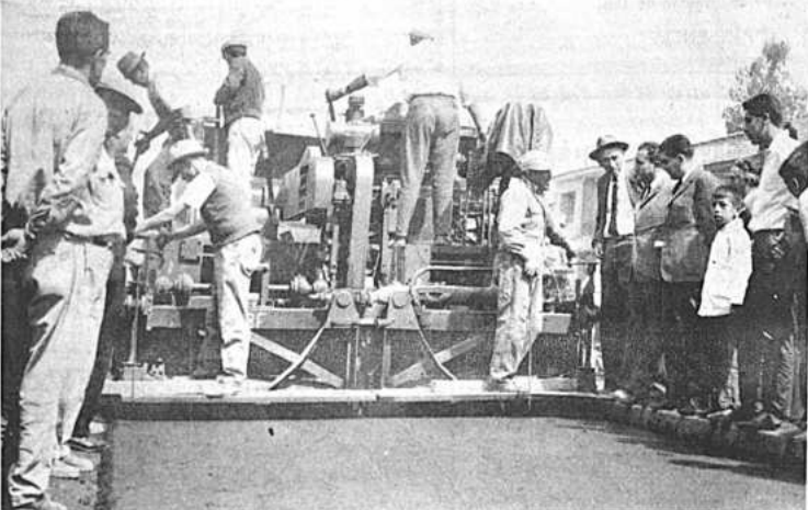
Maquinaria pesada de la Corporación Boliviana de Fomento ejecutando el plan encomendado por el Municipio.
